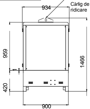
VEDERE FRONTALĂ
