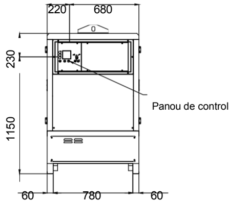
VEDERE SPATE
